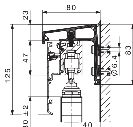
Profilo portante angolare per un piano di scorrimento.
