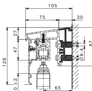
Distanziale profilato (gocciolatoio) per profilo portante angolare per un piano di scorrimento.
