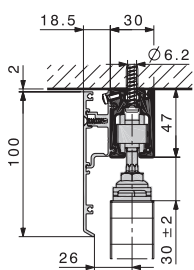
Fissaggio a soffitto o all'architrave della finestra.
