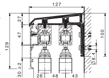
Profilo portante angolare per due piani di scorrimento.
