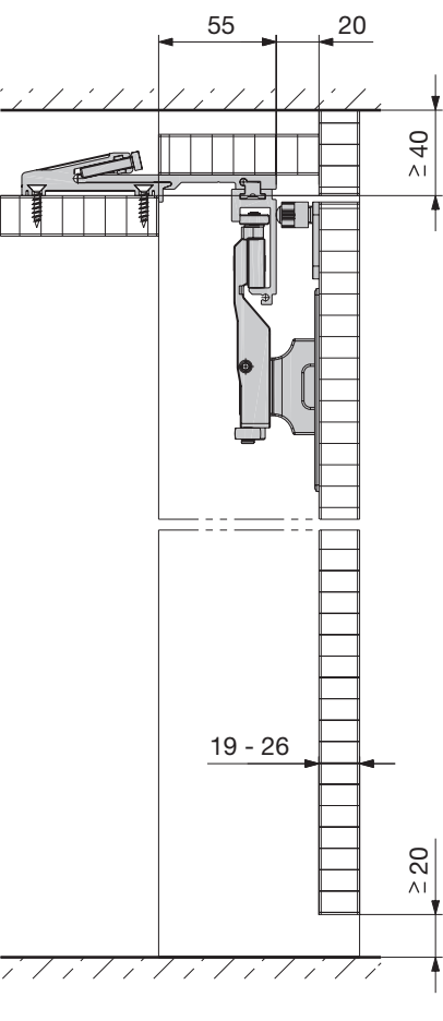
Stropní konstrukce bez nábytkového dna
