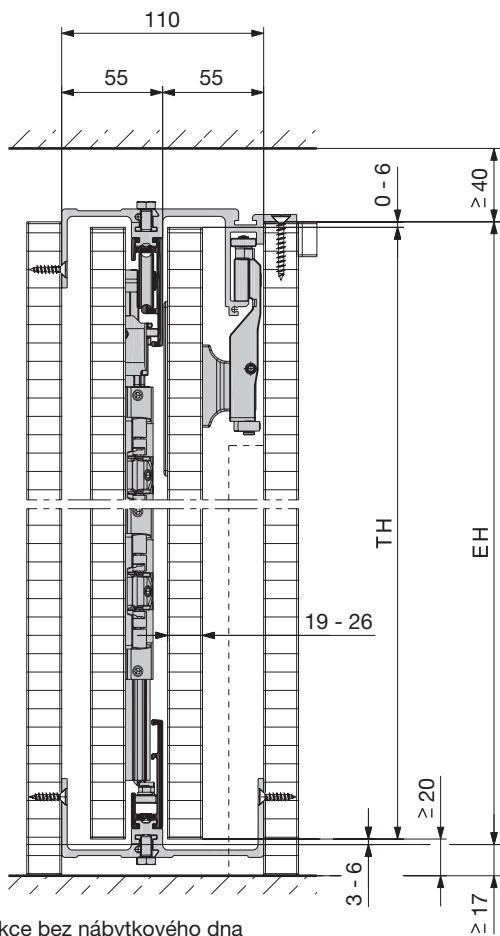
Stropní konstrukce bez nábytkového dna
