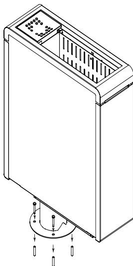
Bild 6 Fixering av Concept R mini combi med stativfot
