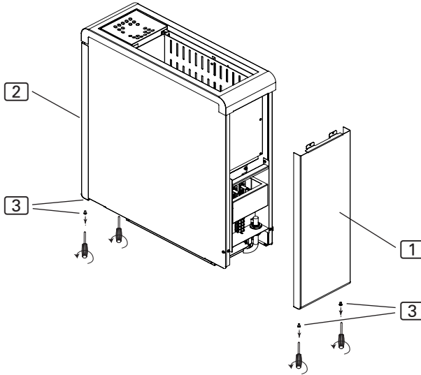
Kuva 10 Katepeltien poistaminen
