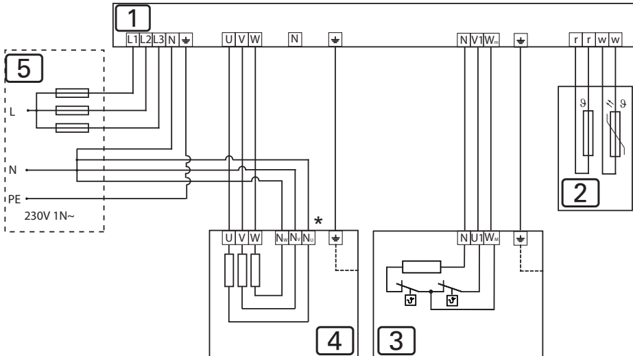
Abb.9 Anschlussplan Concept R mini combi 3,5 kW, 4,5 kW, 6,0 kW und 7,5 kW (CP-RMC-35 / CPC-RM-45 / CR-RMC-60 / CP-RMC-75)
