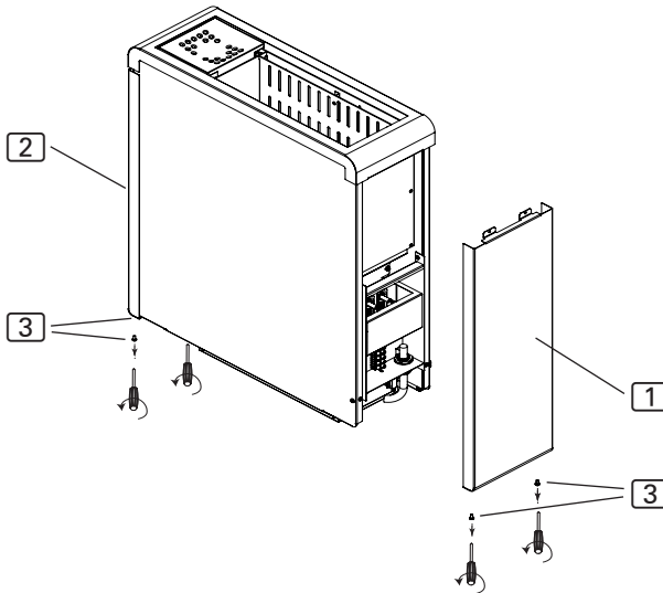
Abb.10 Abdeckbleche entfernen
