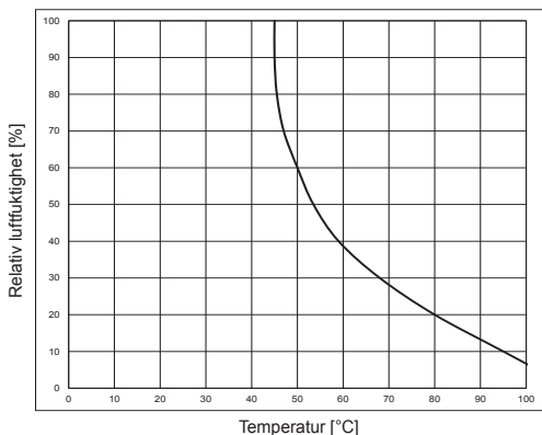
Bild 11 Temperaturkurva/relativ luftfuktighet (enligt EN60335-2-53)
