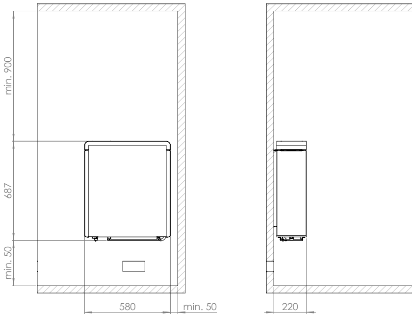
Fig. 1 Distances de sécurité Concept R mini combi 3,5 kW, 4,5 kW, 6,0 kW et 7,5 kW (CP-RMC-35/CP-RMC-45/CR-RMC-60/CP-RMC-75) Dimensions en mm
