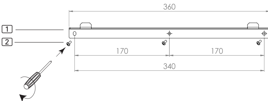
Fig. 2 Barre de montage du Concept R mini combi Dimensions en mm
