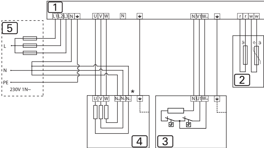
Kuva 9 Liitântäkaavio Concept R mini combi 3,5 kW, 4,5 kW, 6,0 kW ja 7,5 kW (CP-RMC-35 / CPC-RM-45 / CR-RMC-60 / CP-RMC-75)
