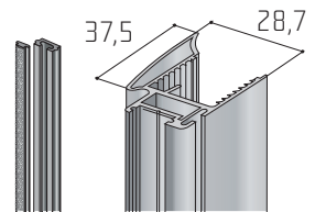
Profil S11N a krycí profil
