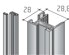
Profil S10N a krycí profil
