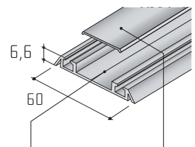
Profil S06 N krycí Profil S06 NN
