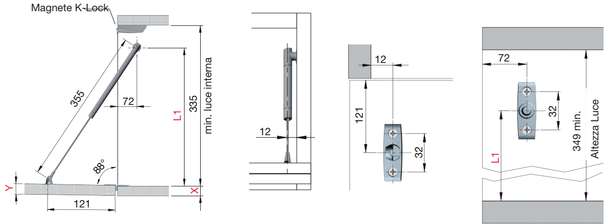
Schema foratura con cerniere Kimana
