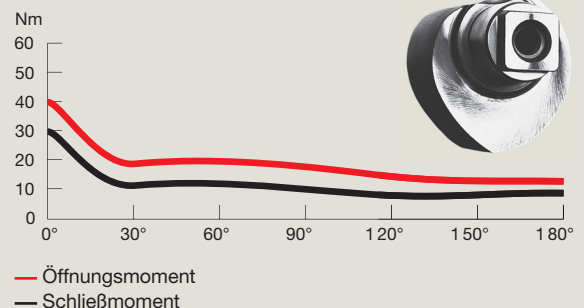
TS 92 XEA B Schließkrafteinstellung Größe EN 4
