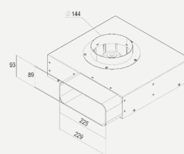
Sockelmotor
