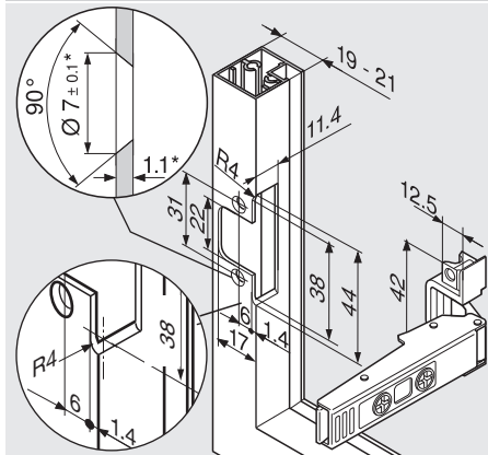
Montaggio a vite (cerniera I piastrina di sup.)
