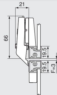
Cerniera centrale CLIP top per alluminio
