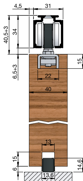
s nosivim čeličnim profilom ME za minimalne visine ugradnje
