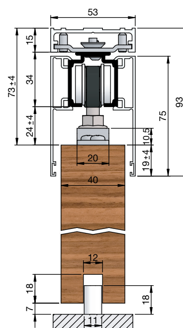
s nosivom priрубnicom, pričvrсна vodilica WT za niše, maska H/G obostrano
