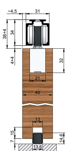
s nosivim alu profilom ME za minimalne visine ugradnje
