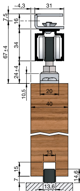
s nosivom priрубnicom, pričvrсни kutnik za niše zidna montaža
