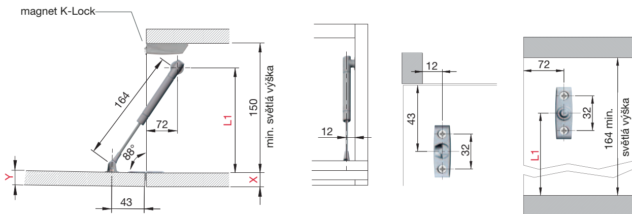
nákres vrtání s miskovými závěsy bez Push to Open (otevřít stisknutím)
