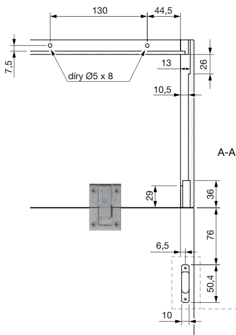
Plánek vrtání zadní stěna
