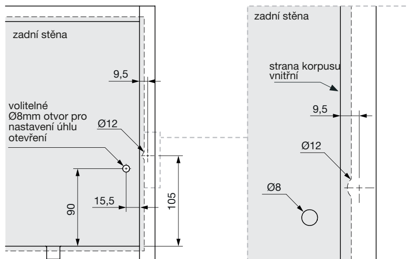
Plánek vrtání zadní stěna
