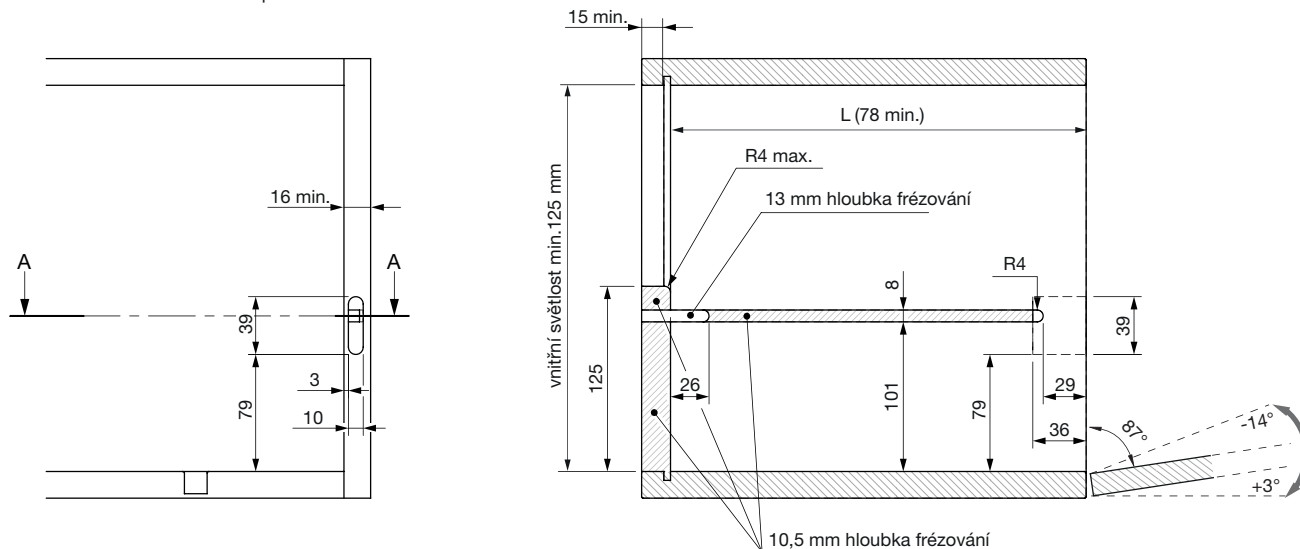
Plánek vrtání na straně korpusu
