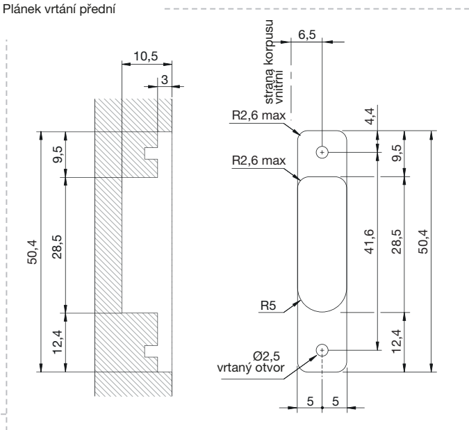
Plánek vrtání přední
