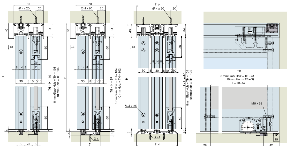
Einbaubeispiel
