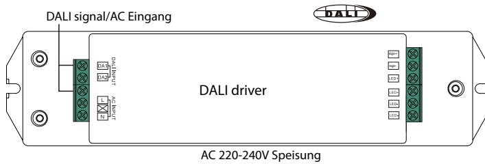
AC 220-240V Speisung
