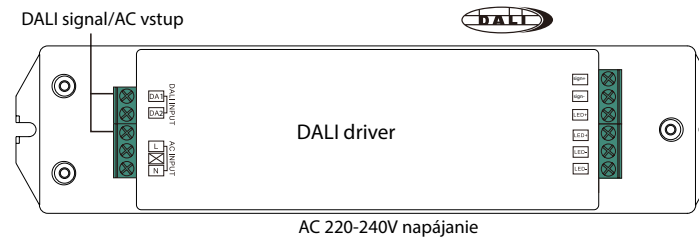
AC 220-240V napájanie
