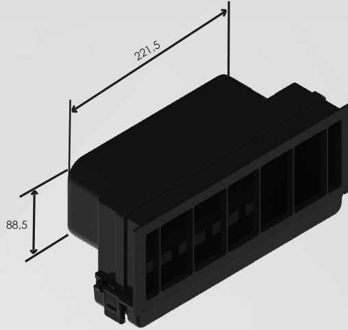
Maße Rückwandstutzen
