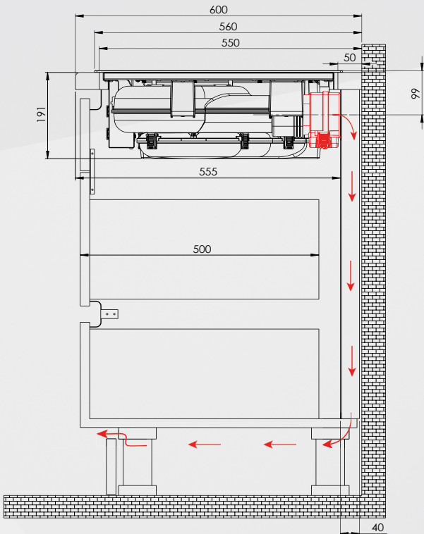
Seitenansicht
