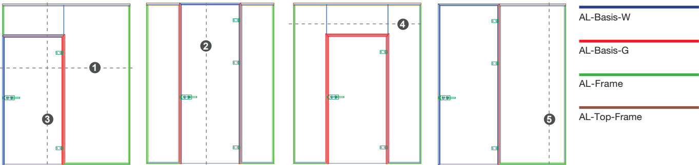
Basis Horizontalschnitt
