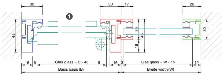
Basis Vertikalschnitt
