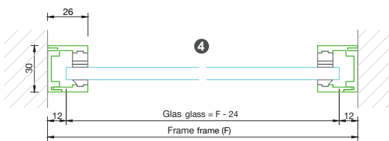
Frame Horizontalschnitt
