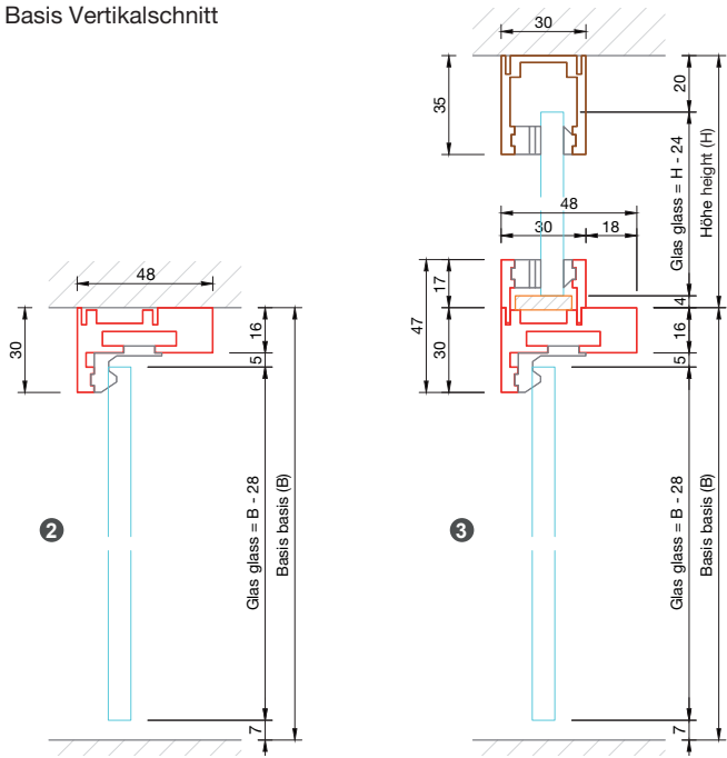
Basis Vertikalschnitt
