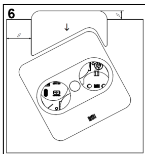
e. Montageschablone optional, für eckige Variante | Mounting template optional, for angular variants
