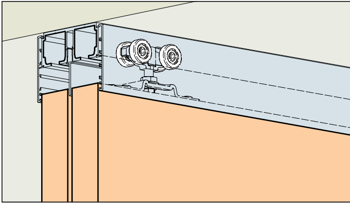
System: Laufschiene obenlaufend, Wand- oder Deckenmontage, für Holztüren bis 100 kg
