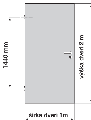
Usporiadanie pri 2 závesoch
