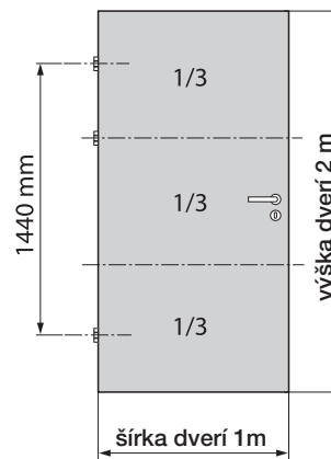
Usporiadanie pri 3 závesoch
