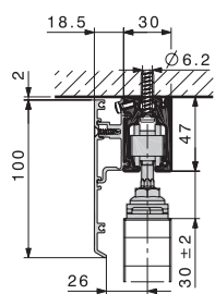
Upevnenie na strop alebo na okenný preklad
