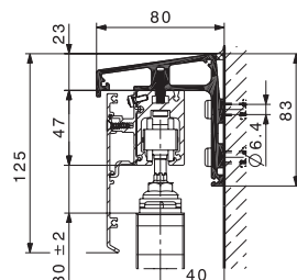
Nosný uhlový profil na úroveň jednej pojazďovej koľajnice
