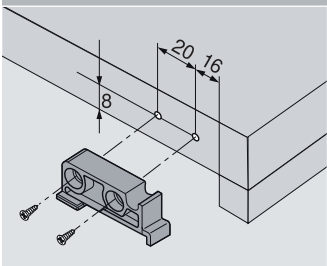
Montaža natičnog držača
