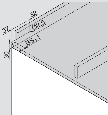
Foratura per piastra di montaggio
