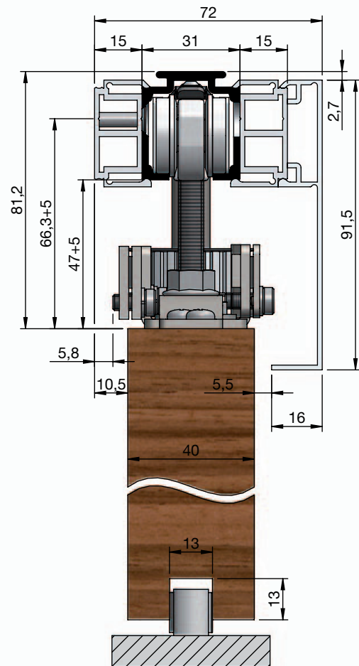
mit Synchronbeschlag, Abstandsprofilen und Blende
