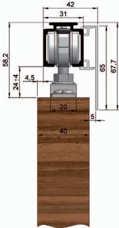
mit Abstandsprofil und Blende
