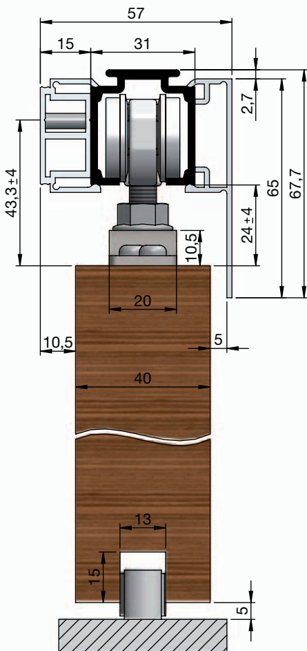
mit Abstandsprofil und Blende
