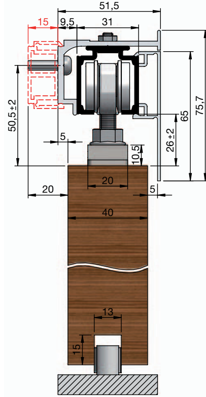
mit Synchronbeschlag, Abstandsprofilen und Blende
