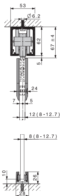
HAWA-Junior 160/GP
