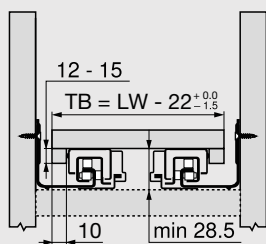
Ripiano estraibile
