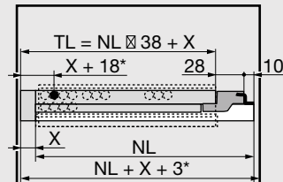
Ripiano estraibile a filo
