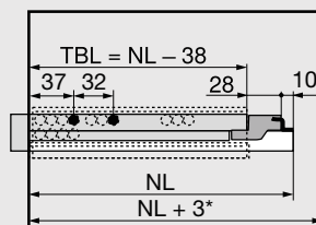
Ripiano estraibile
