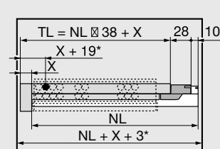
Ripiano estraibile a filo
