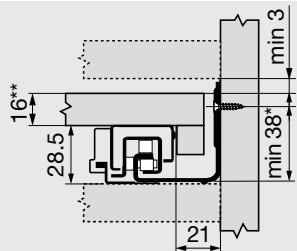
Ingombro nel corpo mobile
