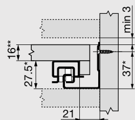
Ingombro nel corpo mobile
