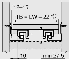
Ripiano estraibile
